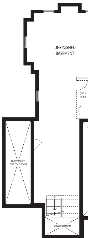
BASEMENT PLAN, STYLE 'B'
